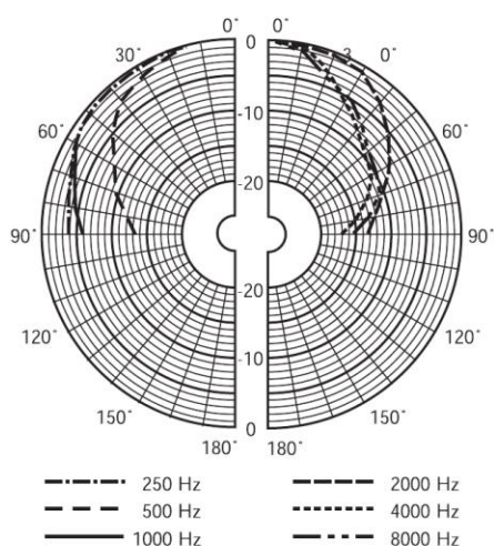
Charakterystyka kierunkowości (pomiar szumem różowym)
