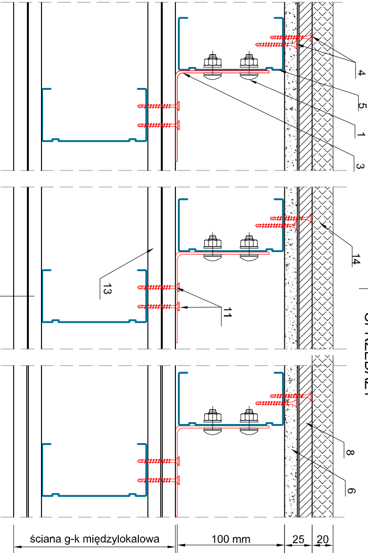
RZUT POZIOMY
