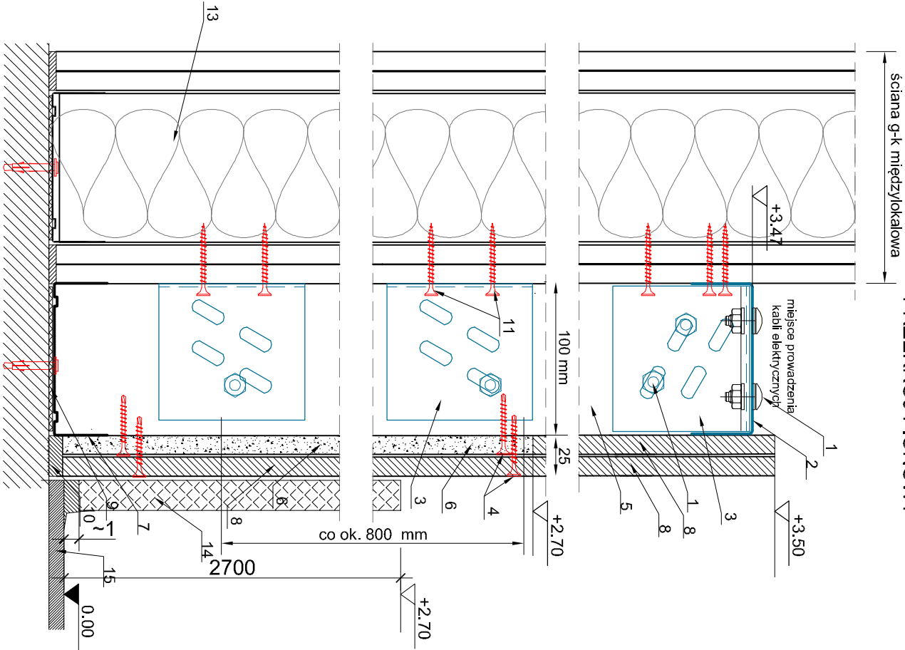
PRZEKRÓJ PIONOWY
