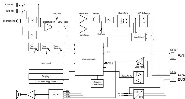
Rys. 1: Schemat elektryczny
