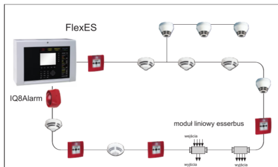
Schemat pętli dozorowej :
