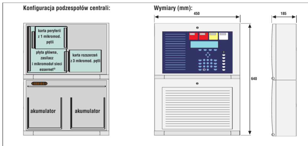
Konfiguracja podzespołów centrali i wymiary
