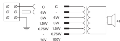
Schemat połączeń
