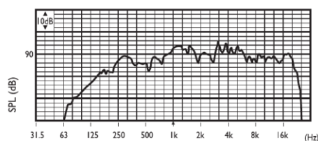
Pasma przenoszenia
