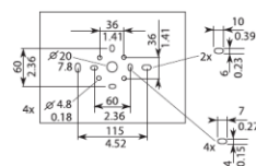
Wymiary montażowe w mm
