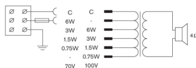
Schemat połączeń
