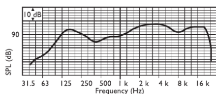
Pasmo przenoszenia
