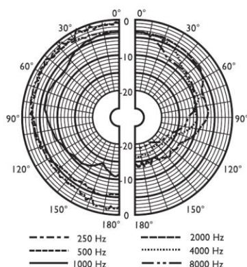
Charakterystyka kierunkowości (pomiar szumem różowym)
