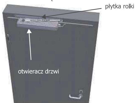
Rysunek 12. Widok od przodu – drzwi „lewe” zamknięte
