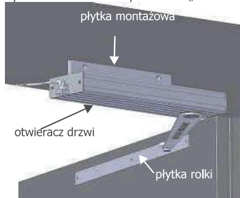
Rysunek 11. Widok od tyłu – drzwi „lewe”
