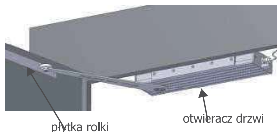
Rysunek 10. Widok od przodu – drzwi „lewe”
