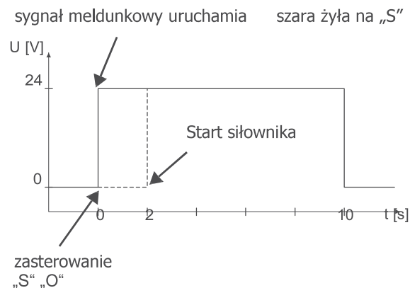
Rysunek 1. Wykres sygnału meldunkowego w kierunku OTWÓRZ
