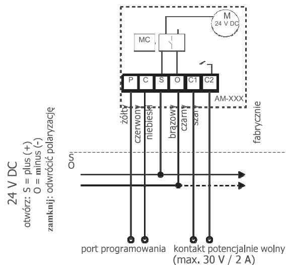
Rysunek 20. Schemat połączeń
