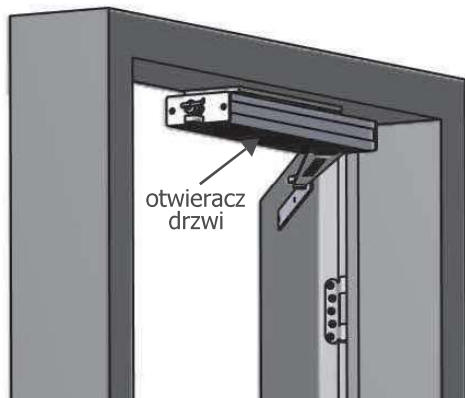
Rysunek 15. Widok od tyłu – drzwi „lewe”
