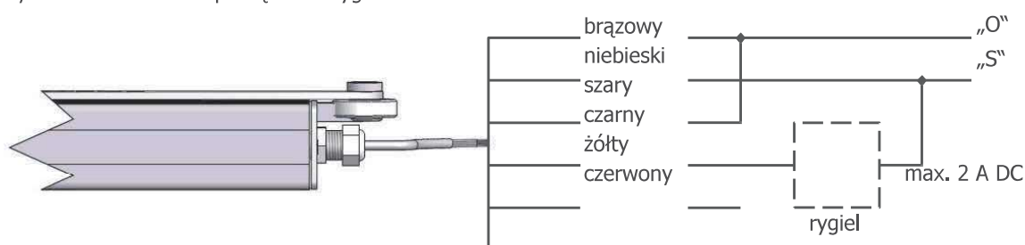
Rysunek 22. Schemat podłączenia rygla
