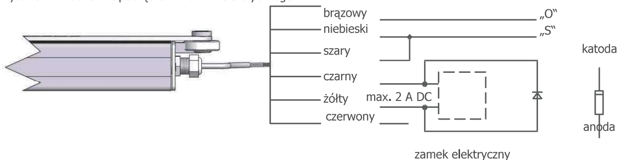
Rysunek 21. Schemat podłączenia zamka elektrycznego
