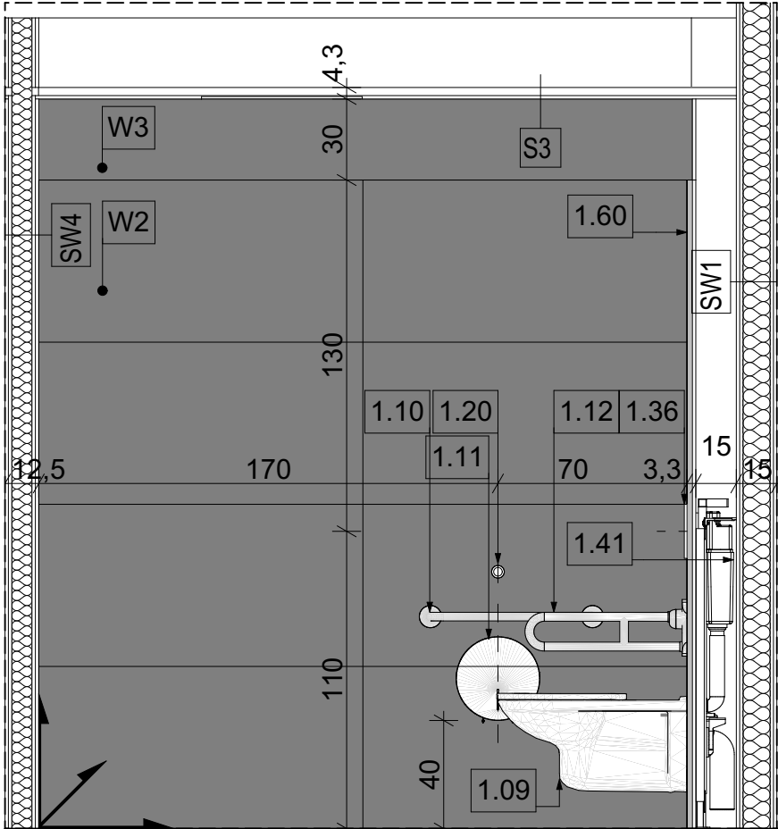
WIDOK A
