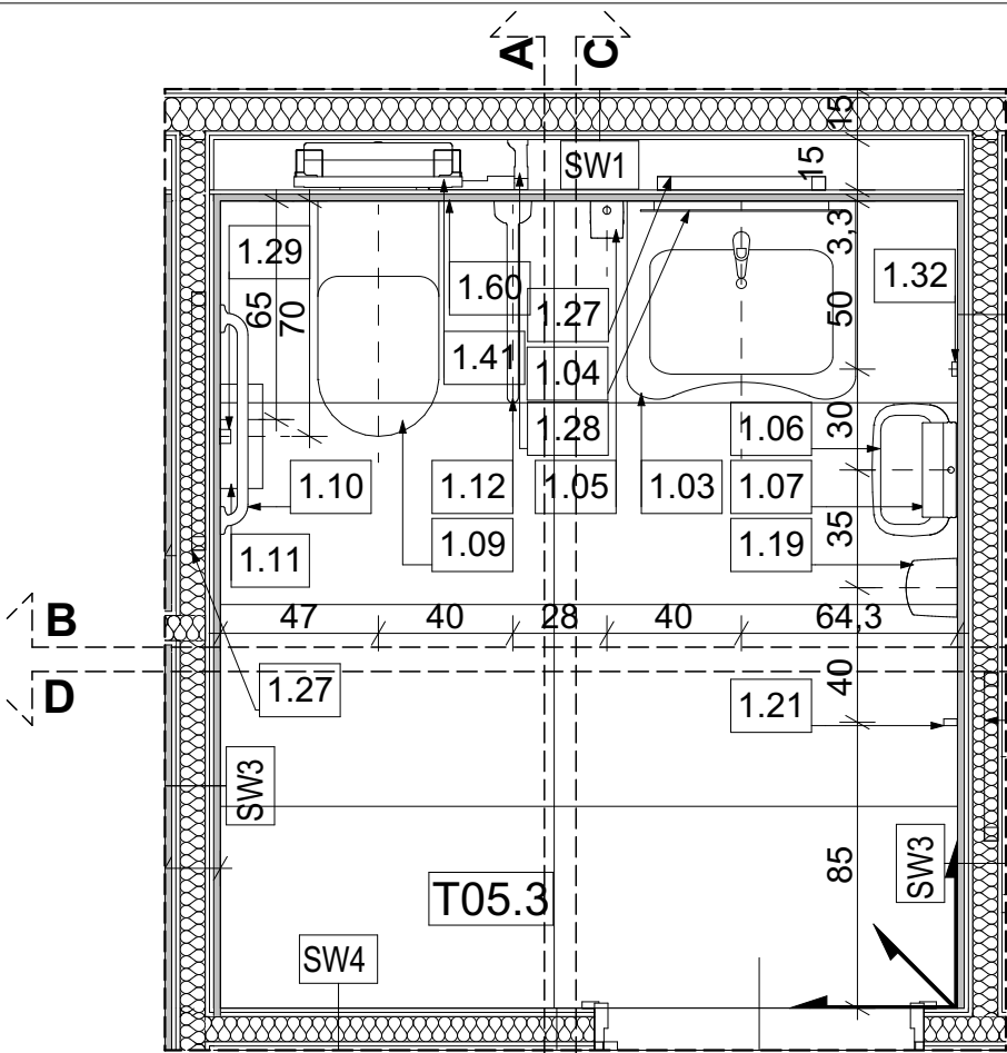
RZUT WĘZŁA SANITARNEGO T05- POSADZKI
