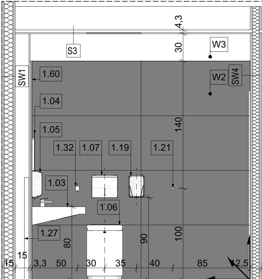
WIDOK C
