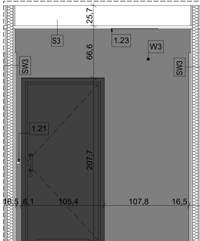
WIDOK D
