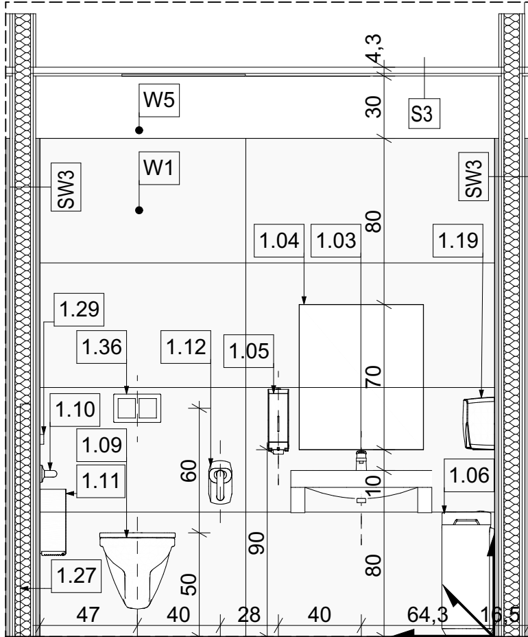
WIDOK B
