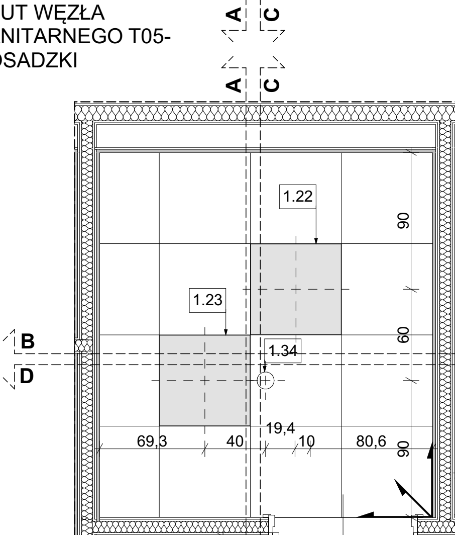
RZUT WĘZŁA SANITARNEGO T05- SUFIT
