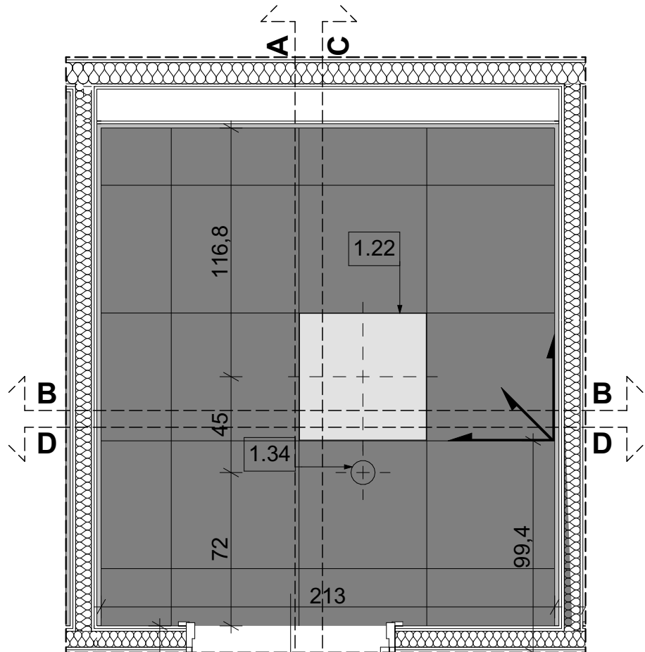
RZUT WĘZŁA SANITARNEGO T04- SUFIT
