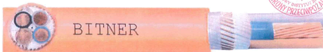
Rys. 4. Budowa kabla (N)HXCH
