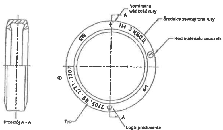
Rys. 5. Uszczelka do złącza
