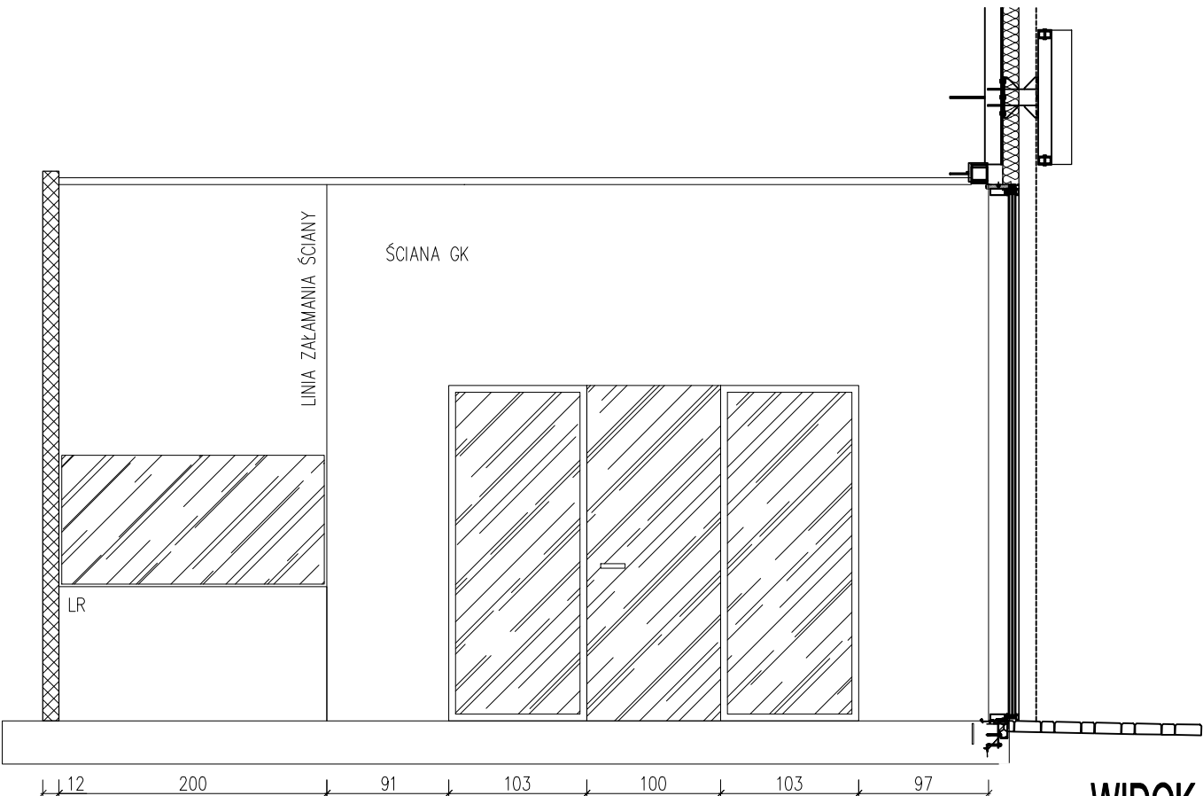
WIDOK B-B
