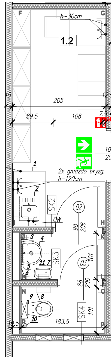
RZUT ZAPLECZA I WC
