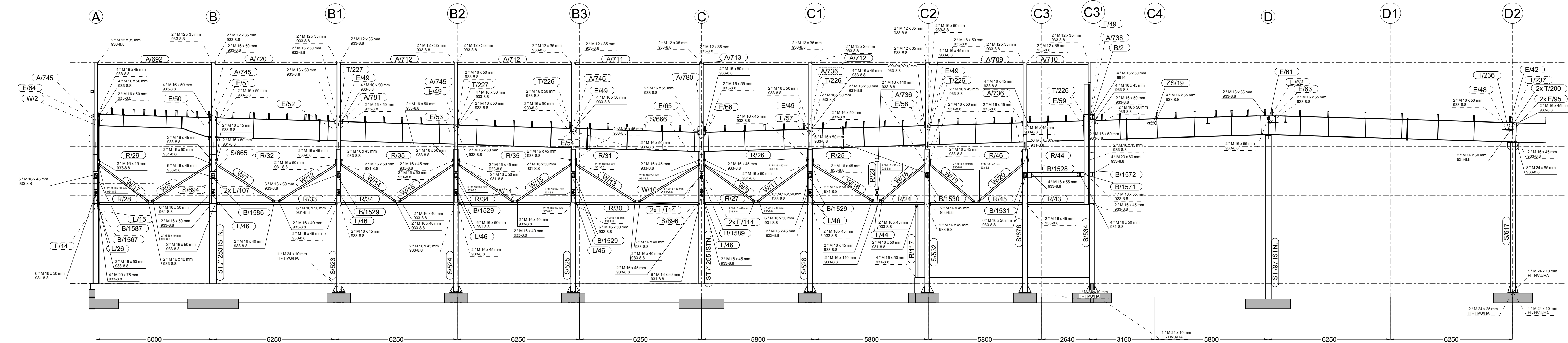
PRZĘKRÓJ W OSI 5/ A-C3' 1:100
