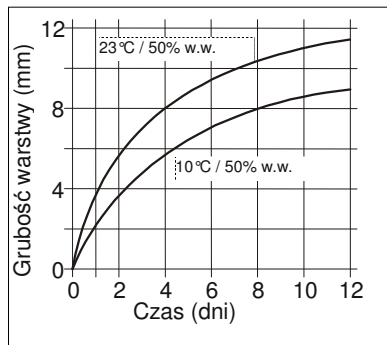
Szybkość utwardzania Sikaflex 221
